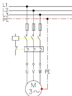
Abb. 10.2.1 – Dreiphasen-Elektropumpen
