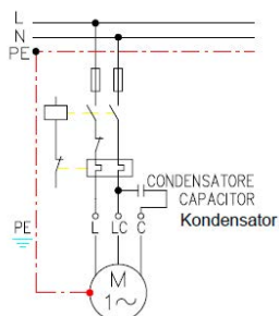
Abb. 10.1.1 – Einphasen-Elektropumpen
